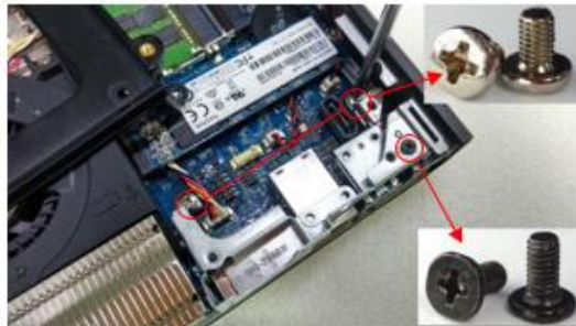
8: Desparafusar e remover o suporte DB9 e antena externa.
