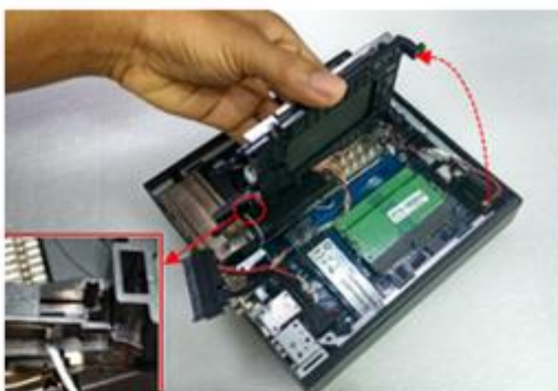
Vire o case de forma em que as travas da antena interna fiquem visíveis.
